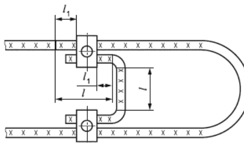
Рисунок 12 - Схема измерения сопротивления электрического контакта
