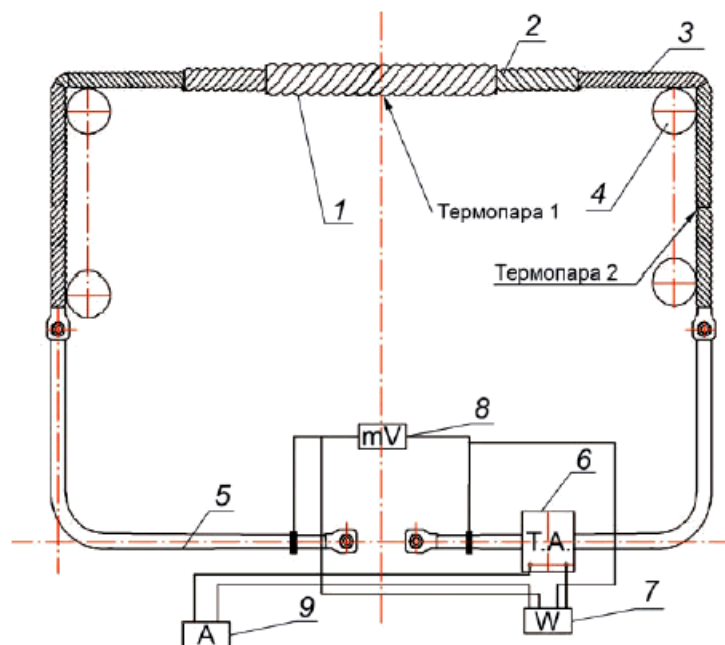
Рисунок 14 - Электрическая схема измерения магнитных потерь в линейной арматуре
