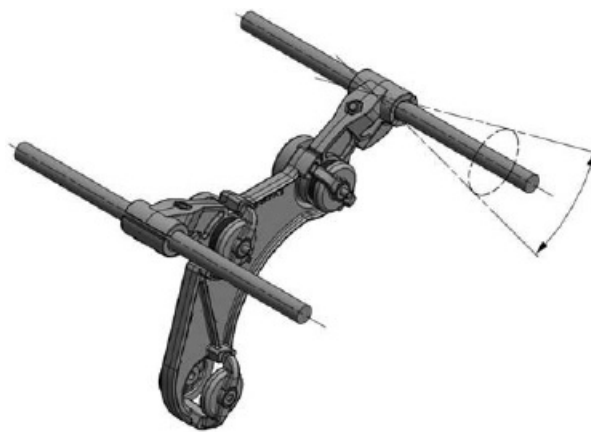
Рисунок 9 - Схема испытаний на вертикальное смещение
